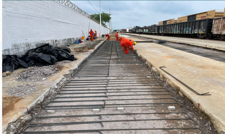
Ampliación de la capacidad de vías Interior, avance: 44.71%
